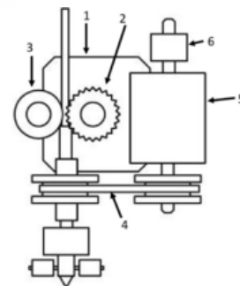
Figura 1: Dispositivo de extrusão de tração direta
